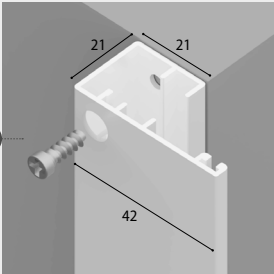
O1 Perçage des coulisses en pose de face Ø 8 mm.
