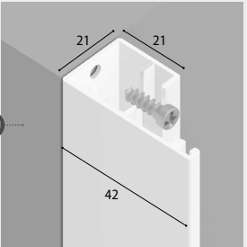
O2 Perçage des coulisses en pose tableau Ø 8 mm.
