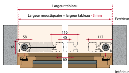
Vue horizontale 2 vantaux
